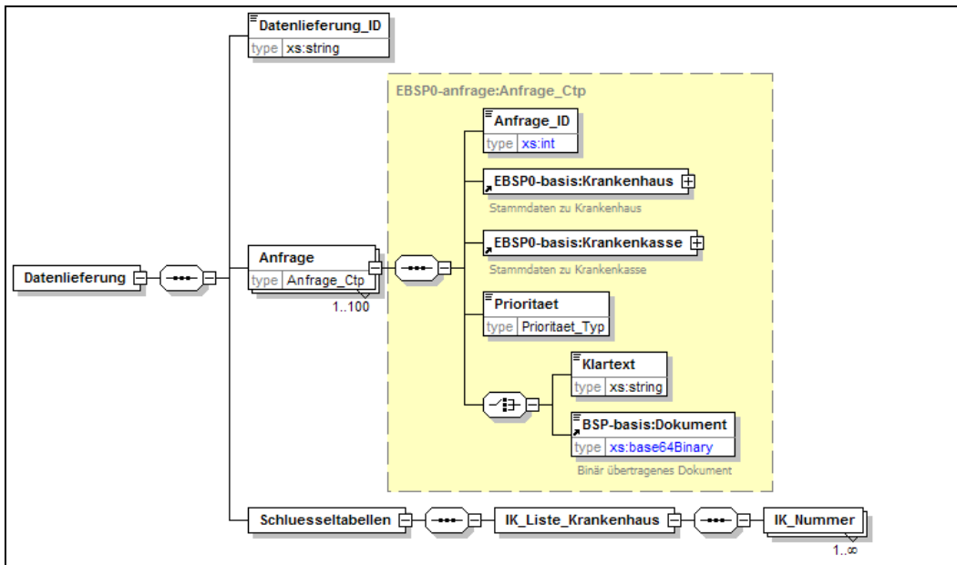
Abbildung 4: Beispiel Schema für ‚Anfrage‘ Nachricht
