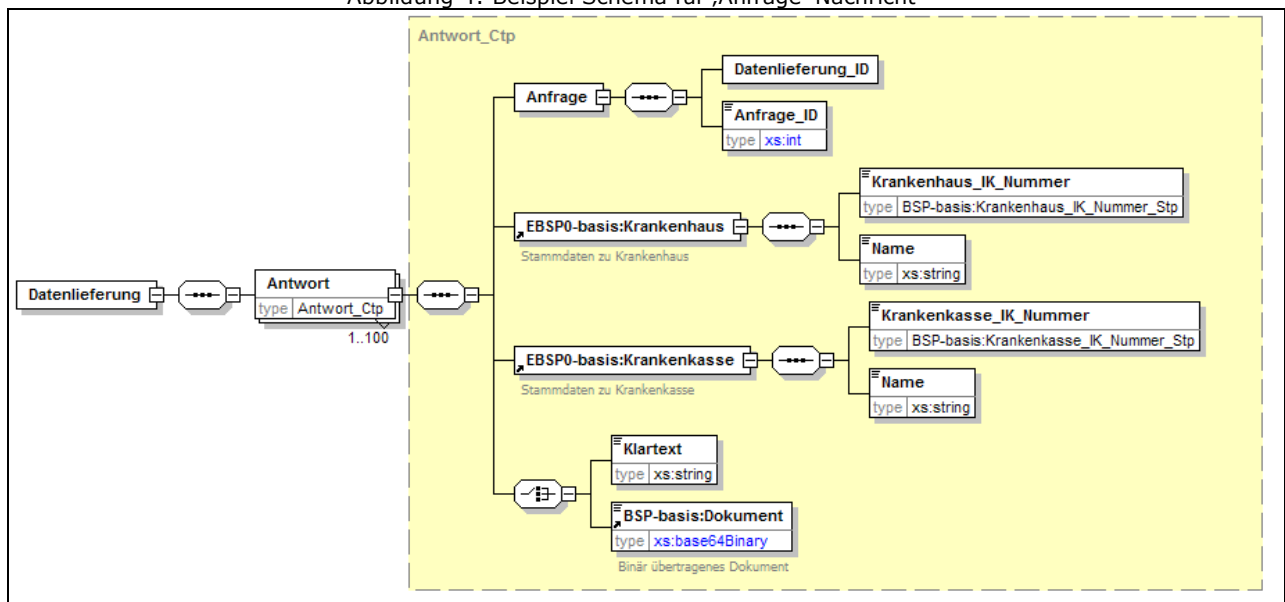
Abbildung 5: Beispiel Schema für ‚Antwort‘ Nachricht
