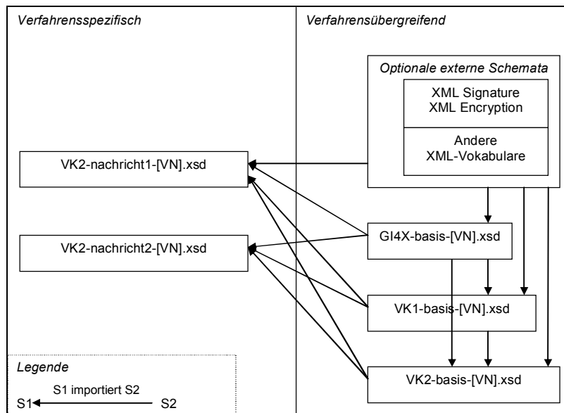
Abbildung 1: Darstellung der Namensraumhierarchie
