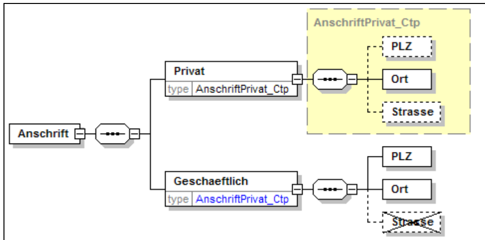
Abbildung 3: Beispiel – Ableitung durch Einschränkung
